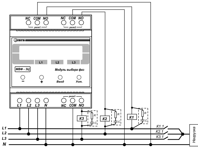
Рис.2. Схема подключения МВФ-3Ц к мощной нагрузке. Необходимо включать параллельно катушке пускателя искрогасящую цепочку R – 51 Ом 1Вт, С – 0,1 мкФ 630 В.
