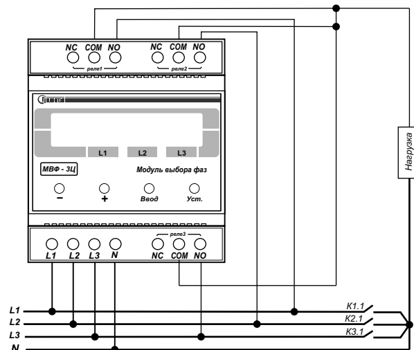
Рис.1. Типовая схема подключения МВФ-3Ц.
